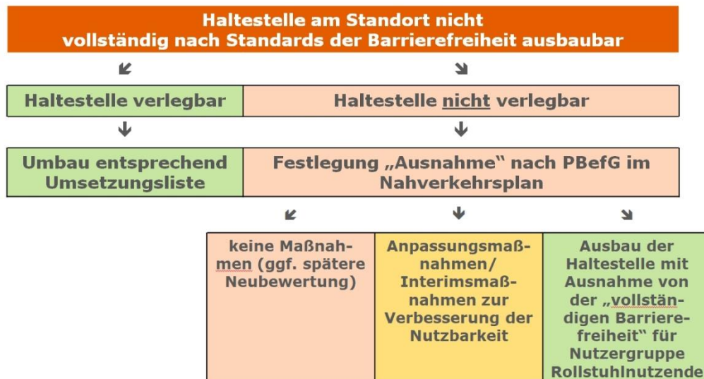
Abbildung 31: Vorgehensweise zum Haltestellenausbau bei problematischen Randbedingungen
