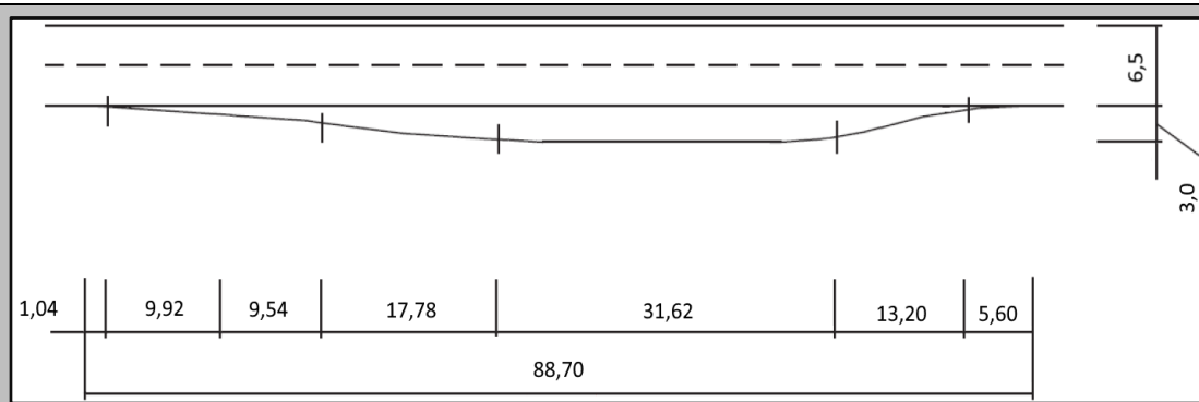
Abbildung 5: Aufgrund der Anfahrtssituation kann eine Halteposition des Busses mit max. 5 cm Höhenunterschied und 5 cm Abstand zur Kante erst ab einer baulichen Länge des Haltebereiches von 88,70 m für Standardbusse bzw. 94,70 m für Gelenkbusse realisiert werden.
